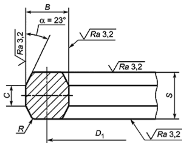
Рисунок 1 - Прокладка металлическая восьмиугольная
