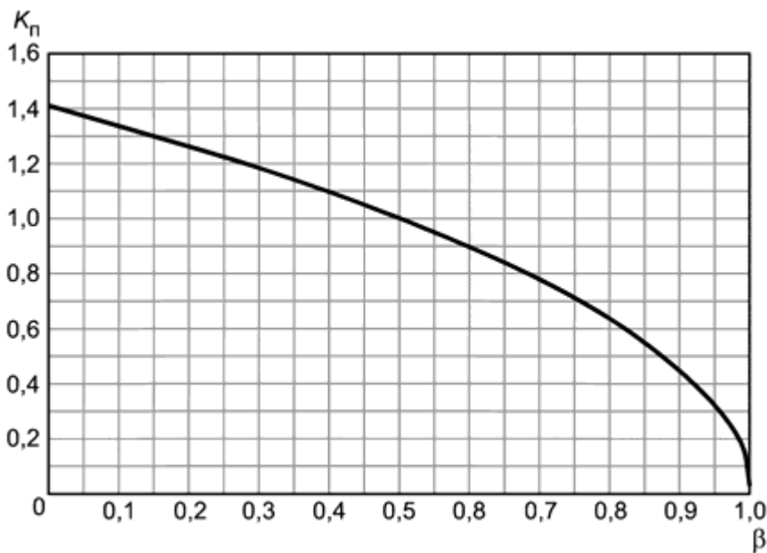
Рисунок Е.1 - Коэффициент K_{II} для несжимаемой жидкости
