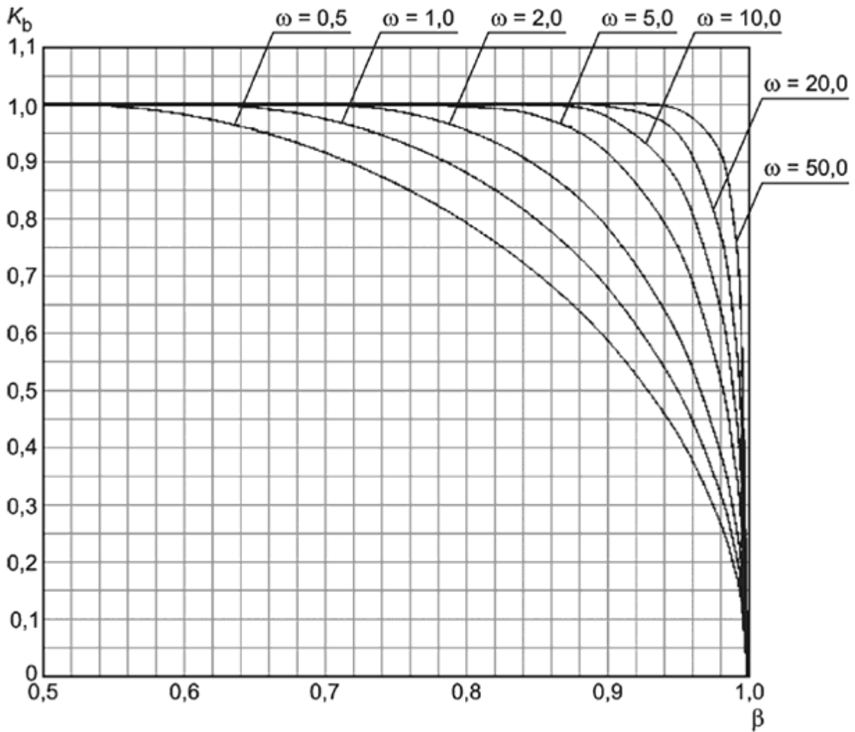
Рисунок Е.6 - Коэффициент K_b для омега-метода
