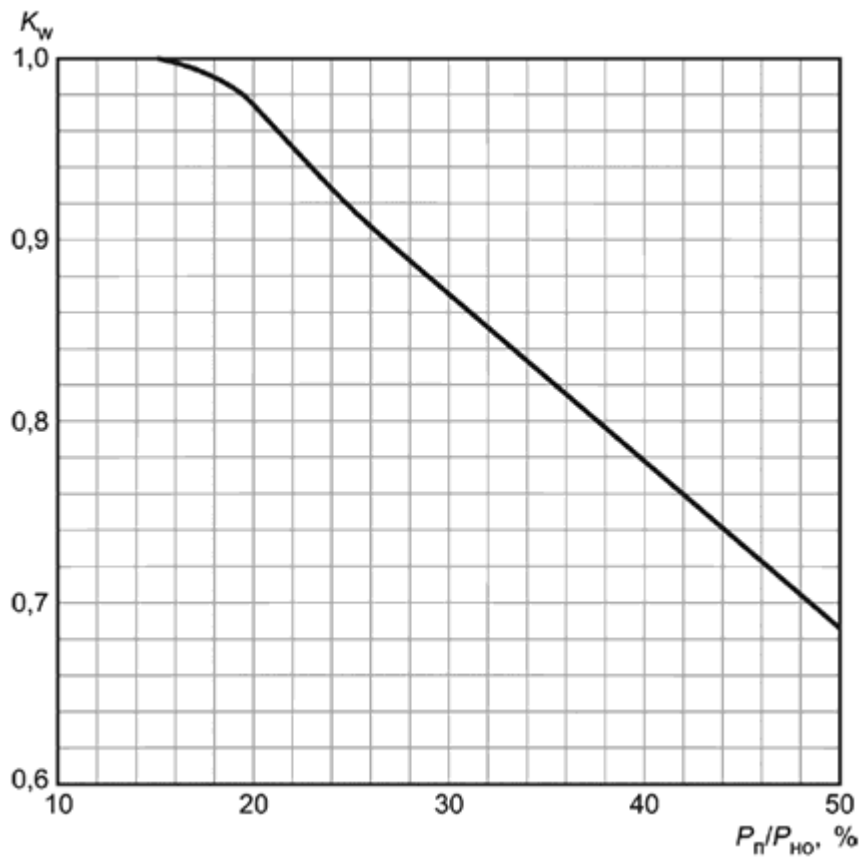
б) При работе клапанов на жидких средах
