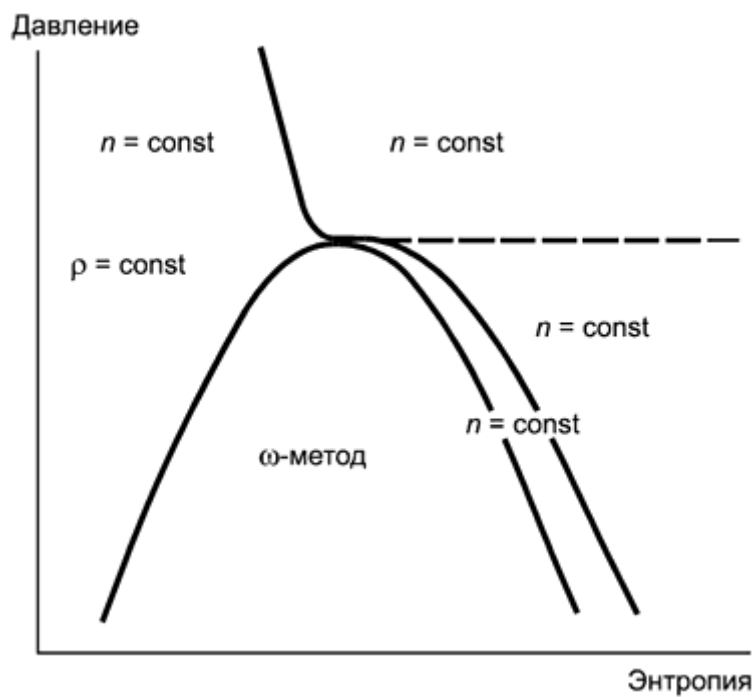
Рисунок Д.1 - Типы фазовых диаграмм и изоэнтропных течений
