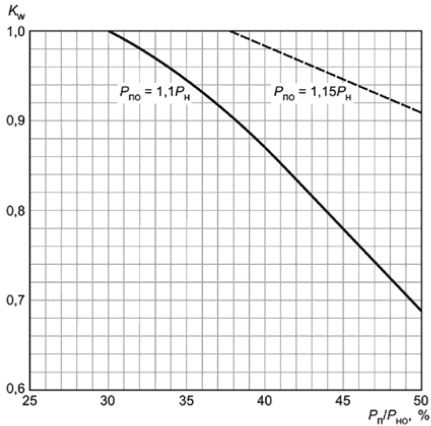
а) При работе клапанов на газообразных средах
