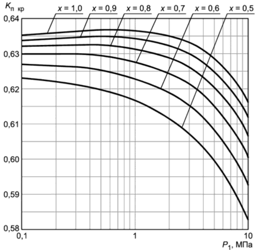
Рисунок Е.9 - Зависимость K_{п кр} = f(P_1) для влажного водяного пара
