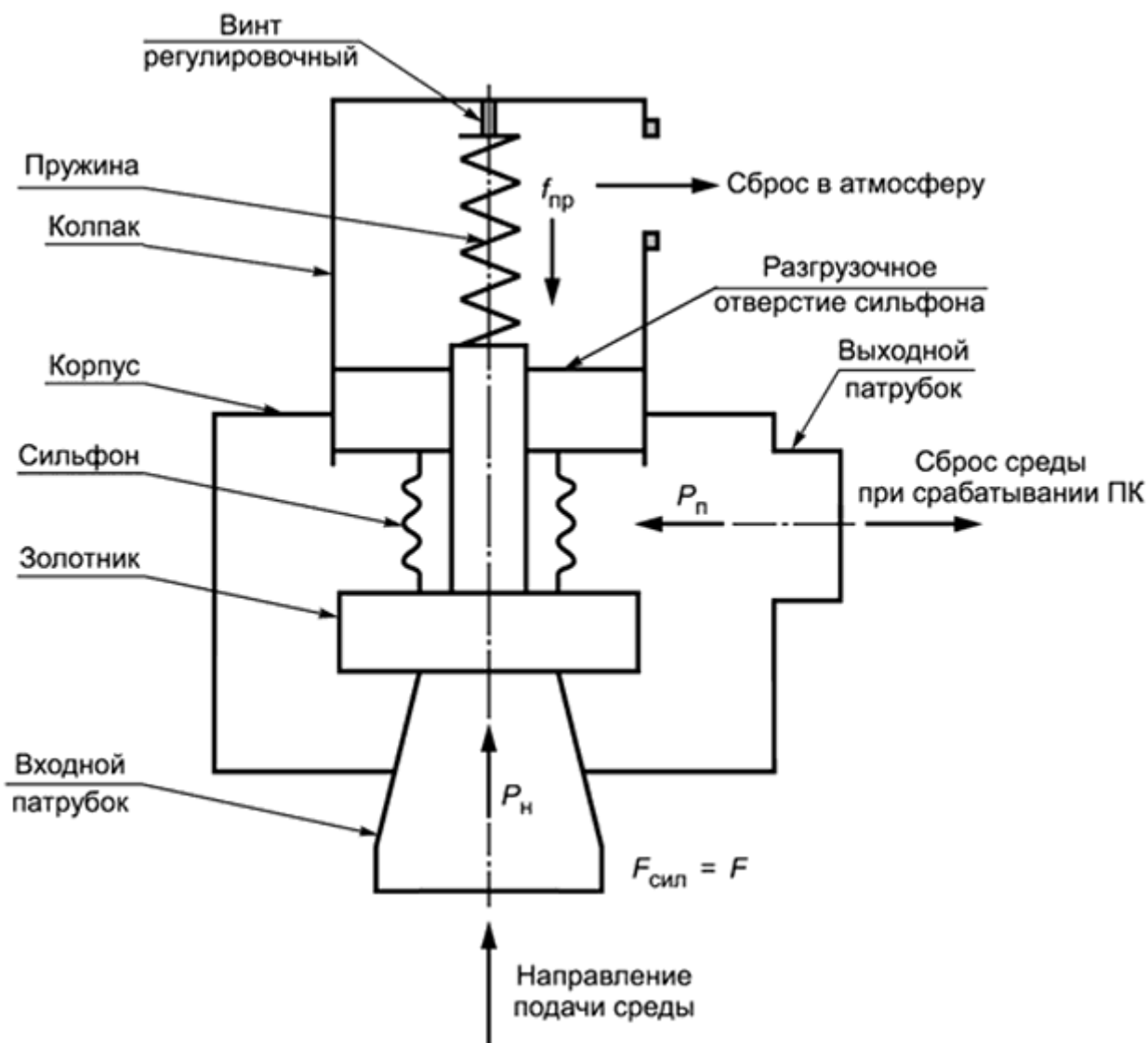
а) С разгрузочным сифоном
