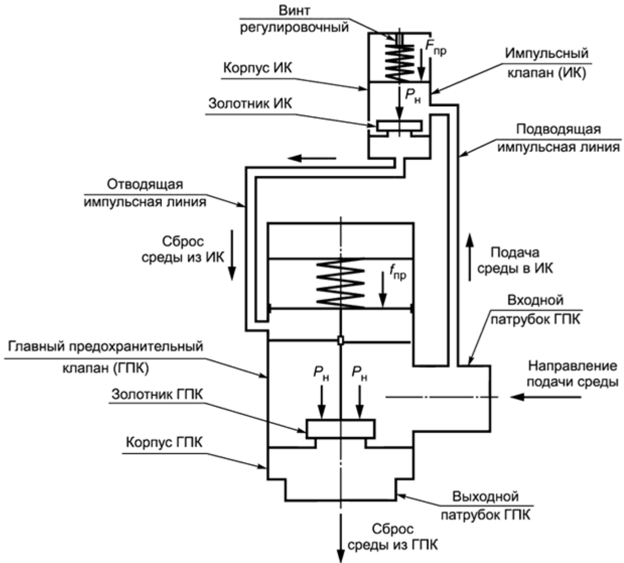
Рисунок В.3 - Импульсно-предохранительное устройство
