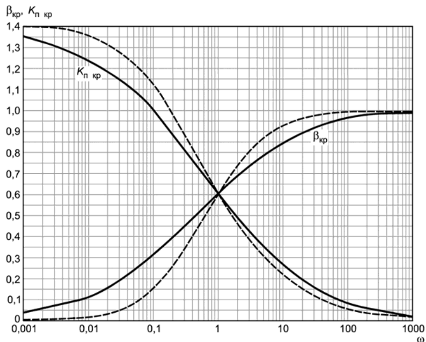
Рисунок Е.2 - Коэффициенты \beta_{кр} и K_{п\ кр} для уравнения постоянного показателя изоэнтропы
