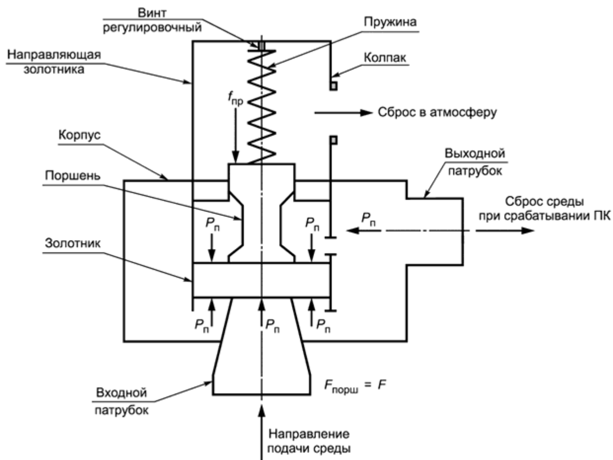
б) Золотник с поршнем
