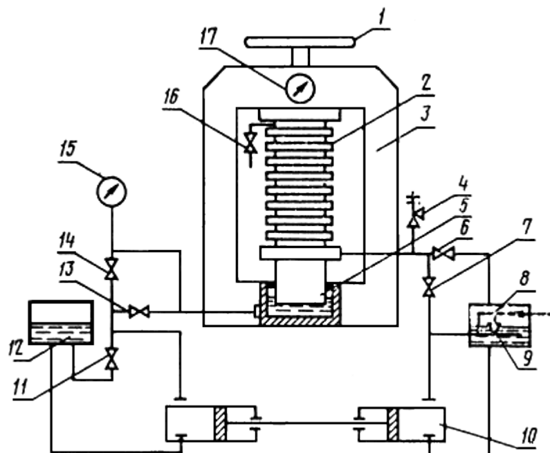
Схема автоклава типа АП-2
